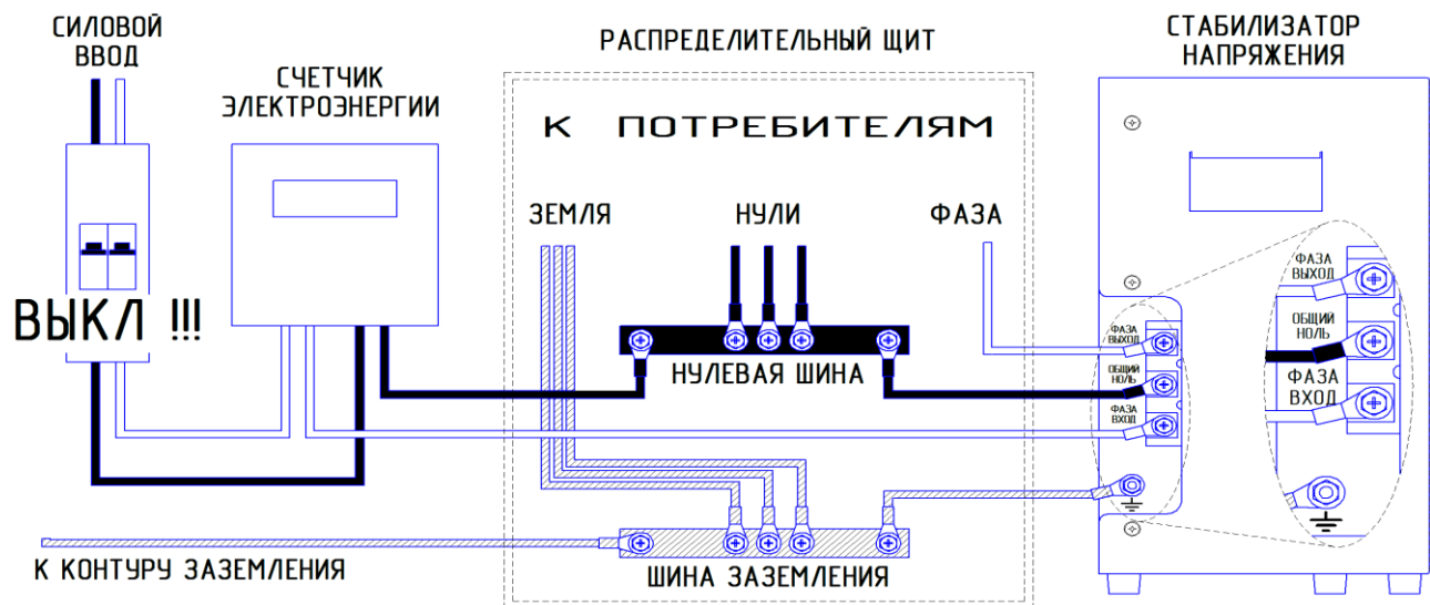
Рисунок 1. Рекомендуемая схема подключения стабилизатора к сети.
