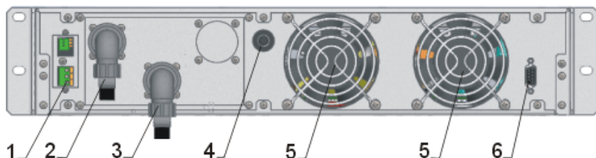
Рис. 1 Задняя панель блока СДП-Т:
