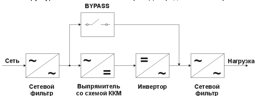
Рис. 2 Структурная схема СДП
