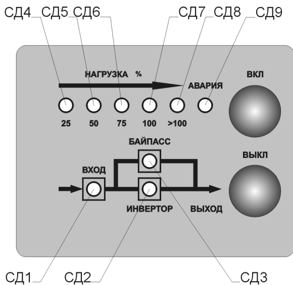
Рис. 3 Панель управления и индикации
