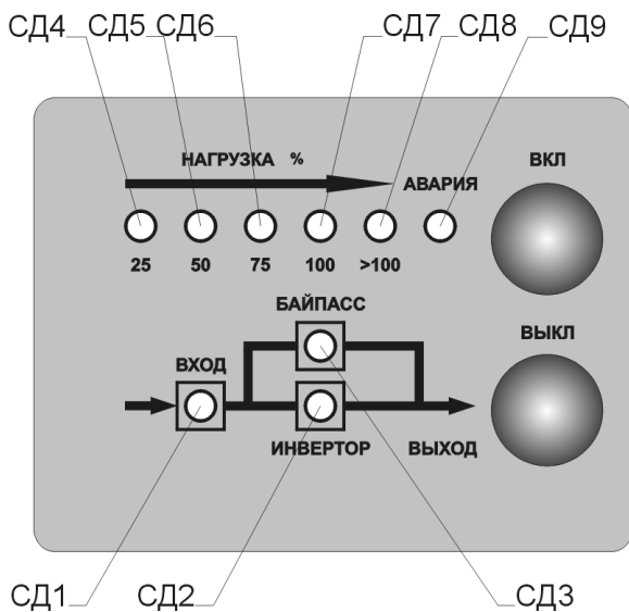
Рис. 2 Панель управления и индикации
