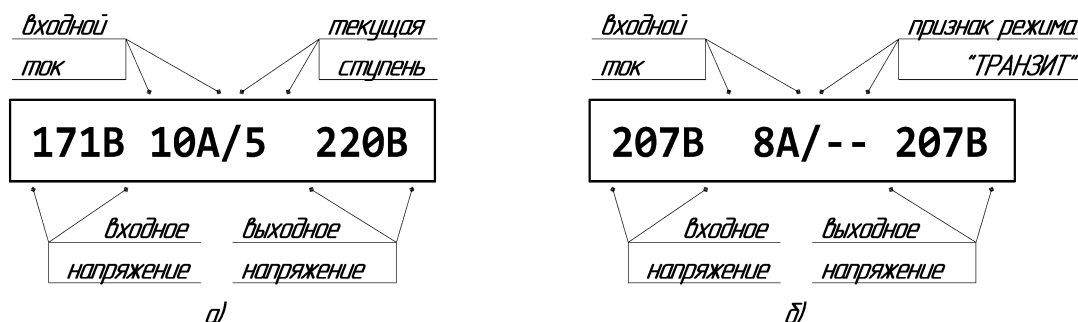
Рисунок 2. Примеры изображений на индикаторе стабилизатора («нулевой экран») а) в режиме «Стабилизация»; б) в режиме «Транзит».
